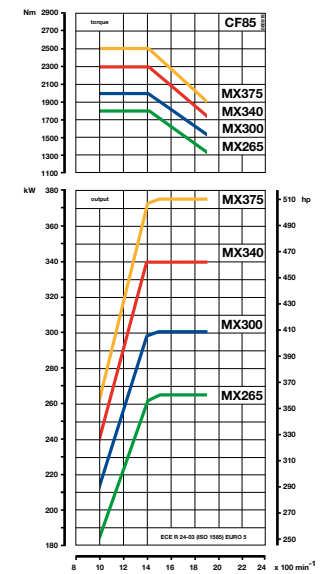
ДВИГАТЕЛЬ PACCAR MX
