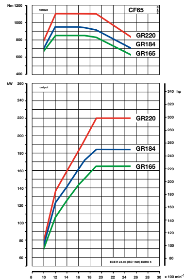
ДВИГАТЕЛЬ PACCAR GR
